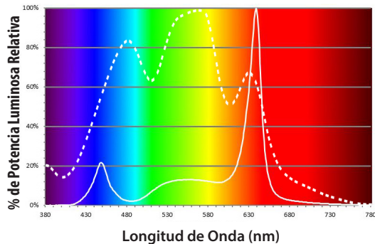
Salida Espectral del TLL Atenuada al 100%
