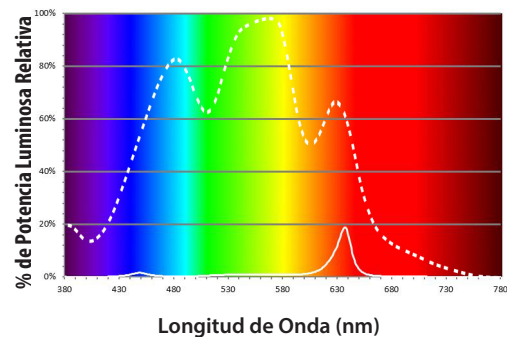
Salida Espectral del TLL Atenuada al 20%
